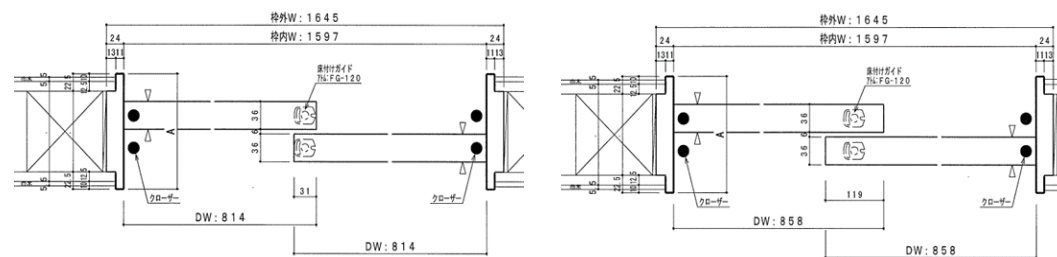
引違い戸(扉重なり31)
