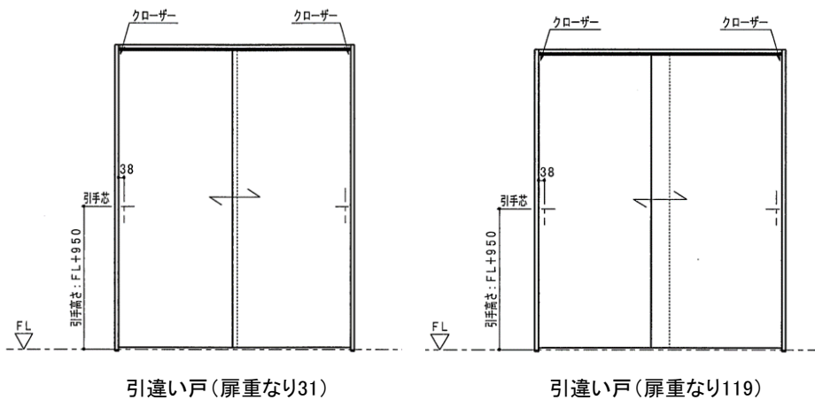
■建具枠セット姿図
