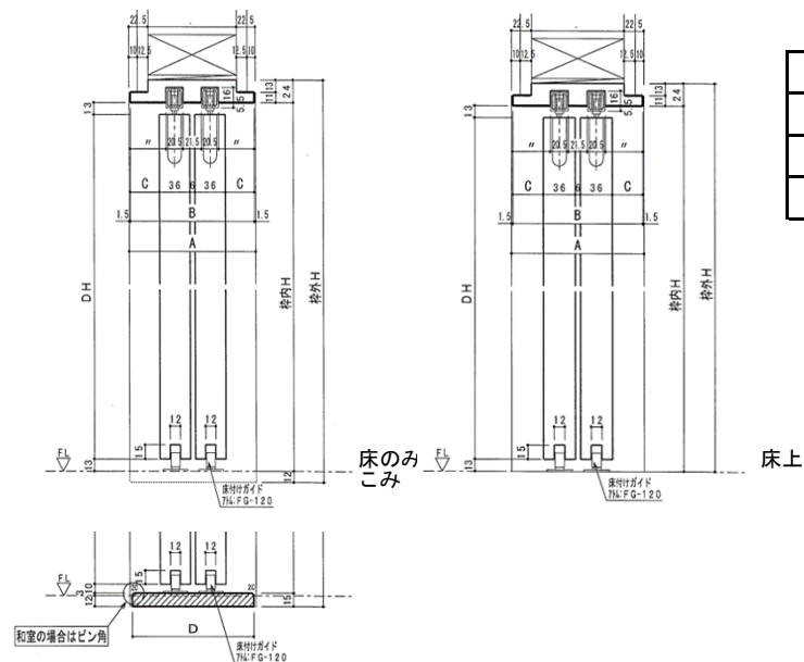
■縦断面図
