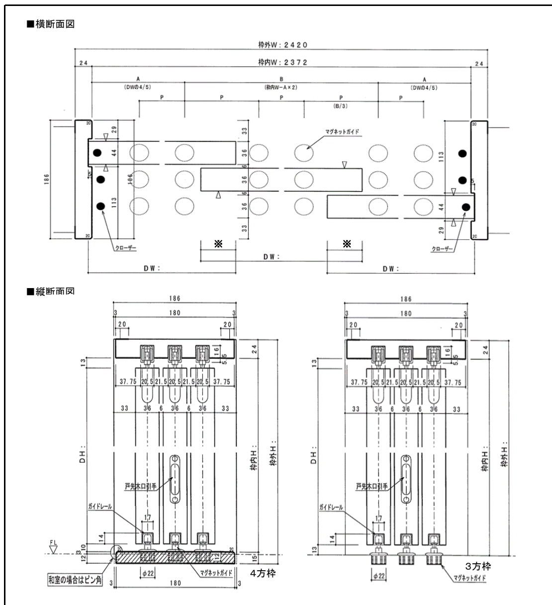
■横断面図・縦断面図
