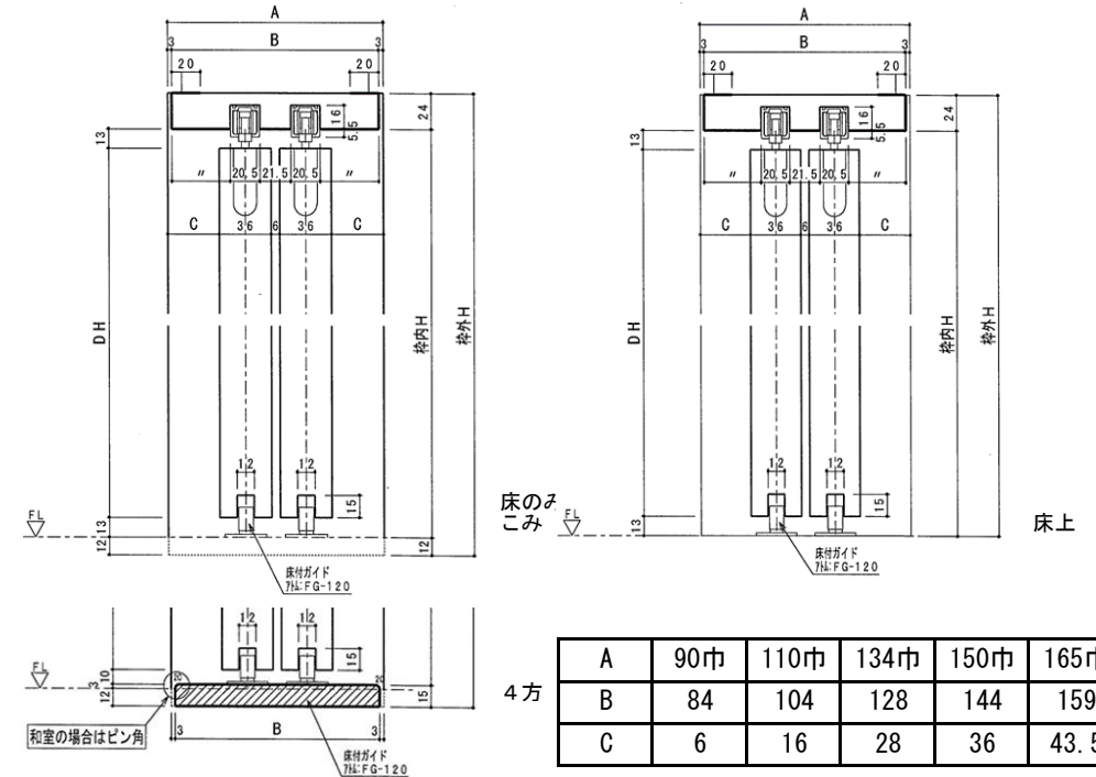
■縦断面図
