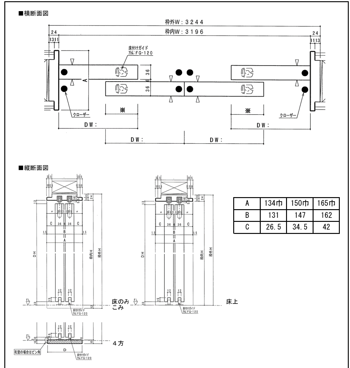
■横断面図・縦断面図
